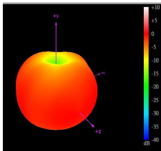
960MHz
