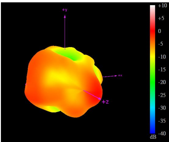
1710MHz
