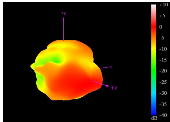
2690MHz
