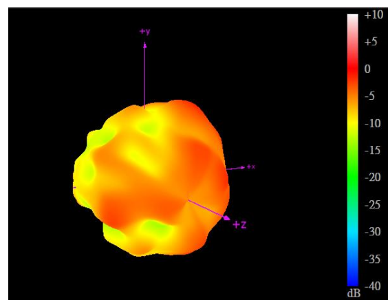
3500MHz
