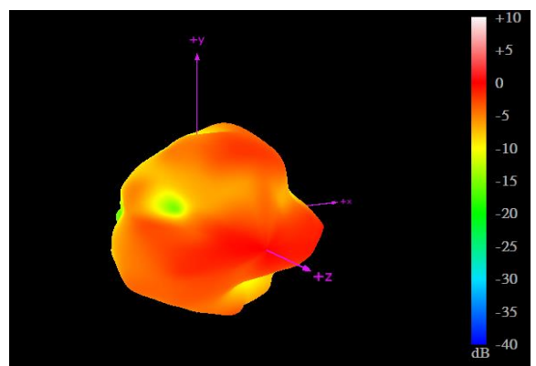
3500MHz
