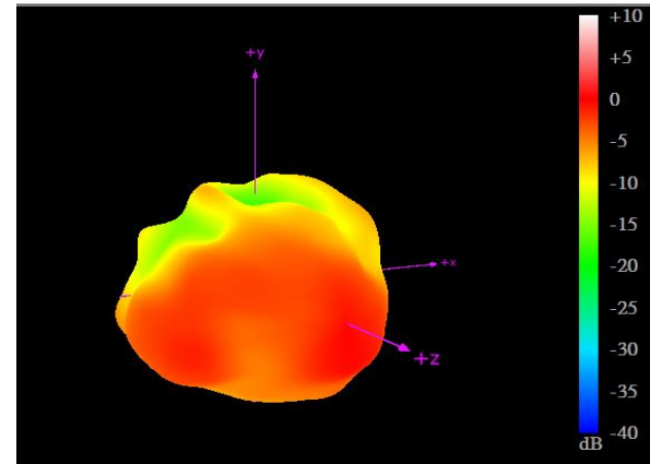
2170MHz
