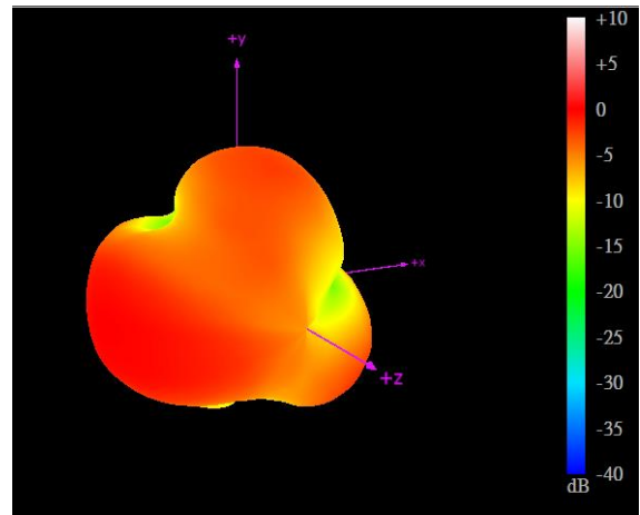
960MHz
