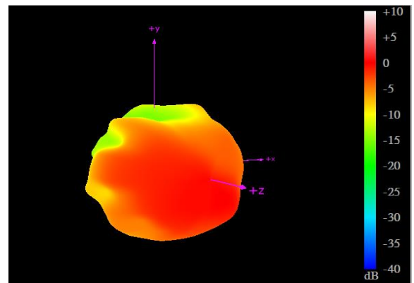
2170MHz
