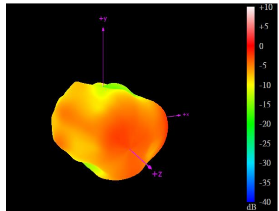
2170MHz
