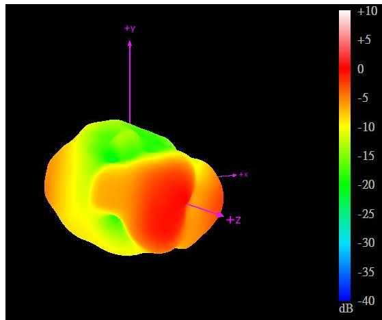
2170MHz
