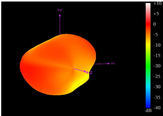
704MHz
