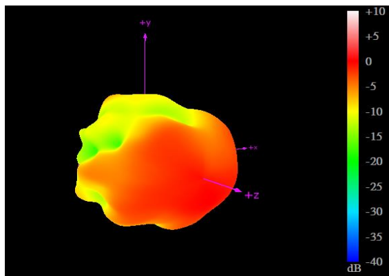
1710MHz
