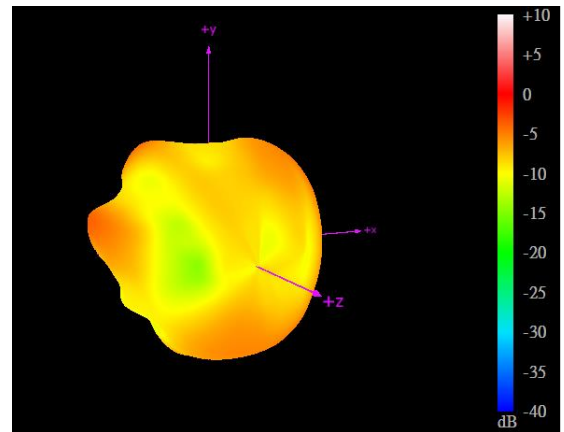
960MHz
