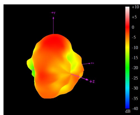
3500MHz
