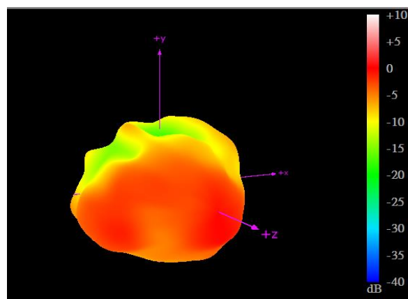
2170MHz
