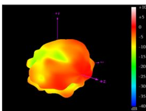
3500MHz
