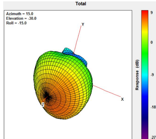
2170MHz
