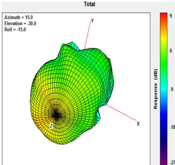
1710MHz
