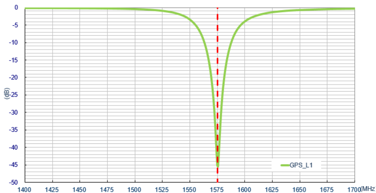
L1 1575MHz
