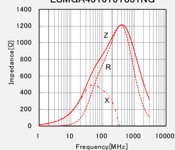
4532 type
