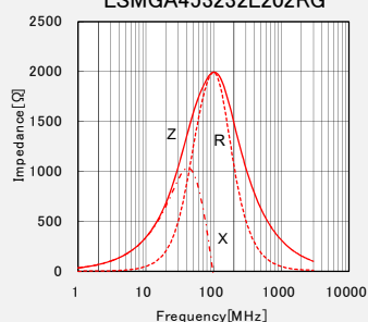
LSMGA453232L202RG
