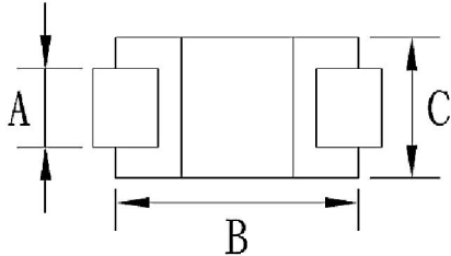
DO-214AC (SMA)
