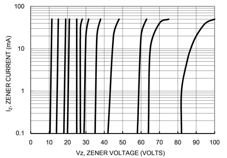
FIG. 7- V_z = 11 - 91 VOLTS
