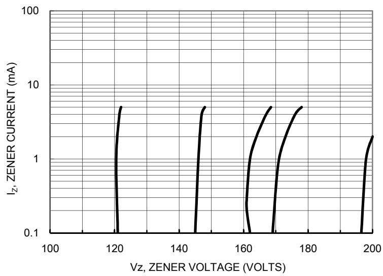
FIG. 8- V_z = 100 - 200 VOLTS
