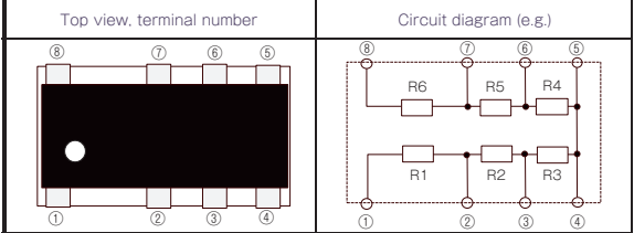
RM11264(11.2mm×6.4mm)
