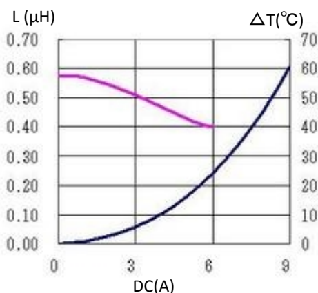
4. 0320CDMCCDS-R56MC
