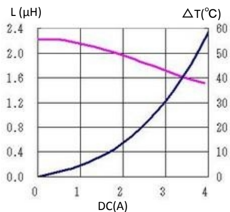
9. 0320CDMCCDS-2R2MC
