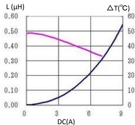
3. 0320CDMCCDS-R47MC
