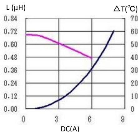
5. 0320CDMCCDS-R68MC
