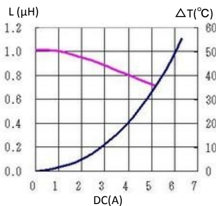
7. 0320CDMCCDS-1R0MC
