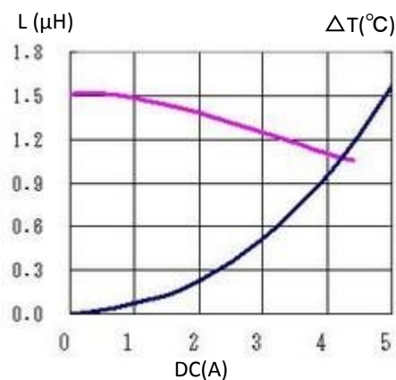
8. 0320CDMCCDS-1R5MC
