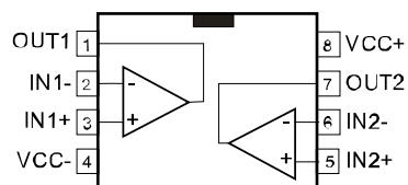
SO8 (TSZ182H)
