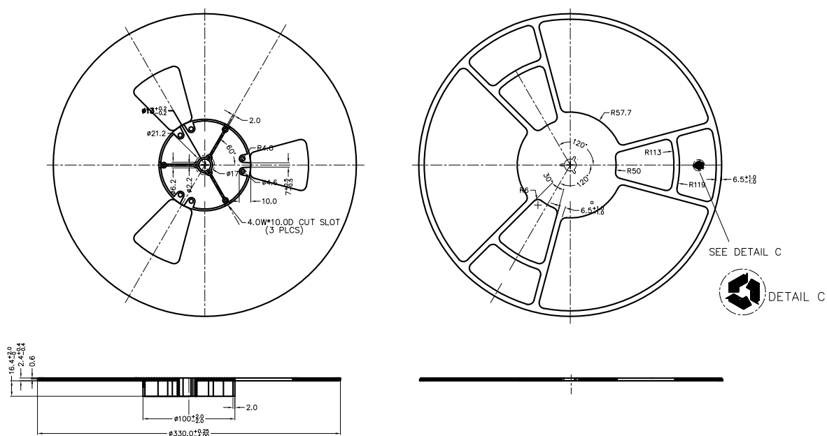
Figure 13. PowerFLAT™ 8x8 HV reel
