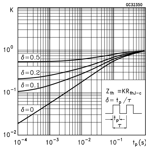
Thermal Impedance
