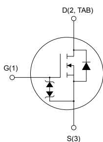
DPAK
