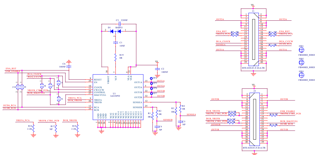
Figure 9. EVL6228-PLUG
