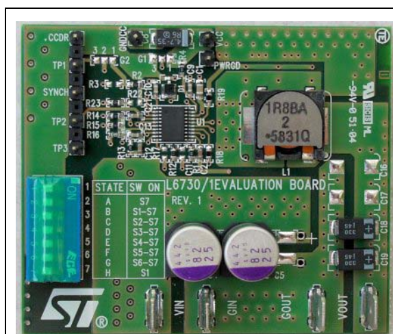
STEVAL-ISA025V1
