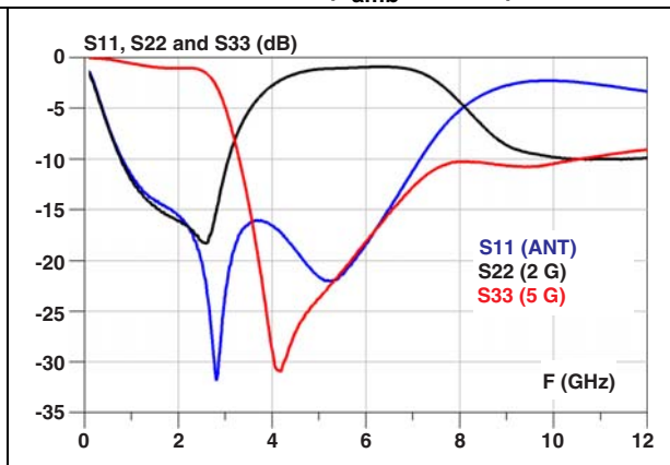
Figure 3. 2 G, 5 G and antenna reflection coefficient (T amb = 25 °C)
