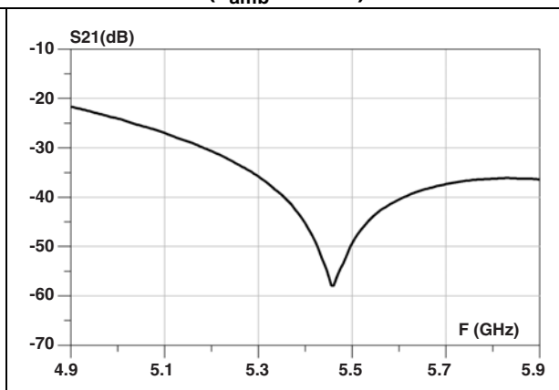
Figure 5. 2 G attenuation in 5 G band (T amb = 25 °C)
