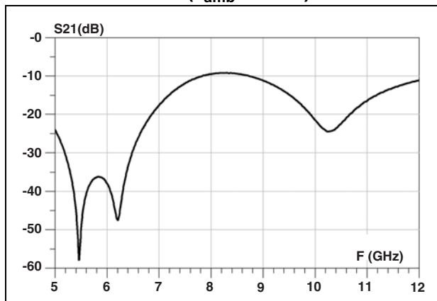
Figure 6. 2 G attenuation in high frequency band (T amb = 25 °C)
