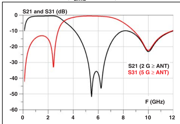
Figure 2. 2 G and 5 G forward transmission (T amb = 25 °C)
