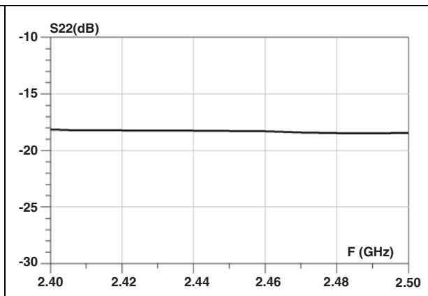
Figure 7. 2 G return loss (T amb = 25 °C)
