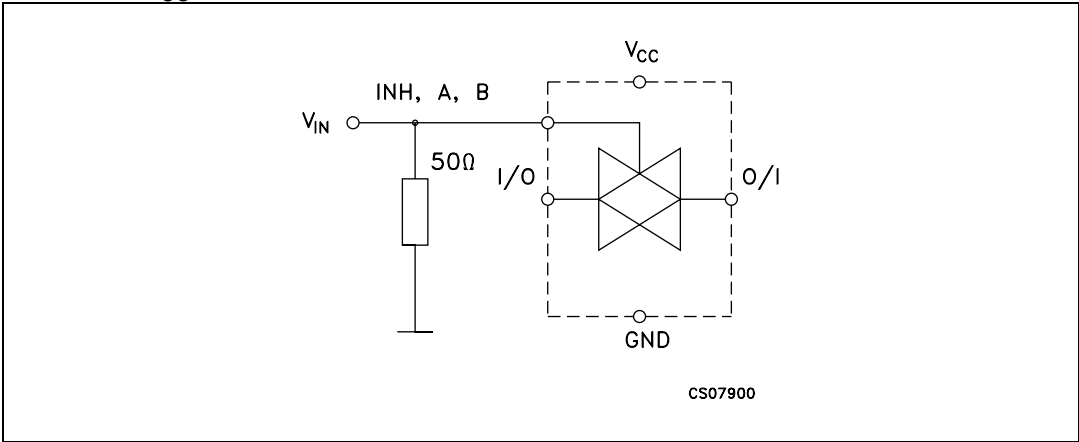
Figure 11. I_{CC} (opr.)
