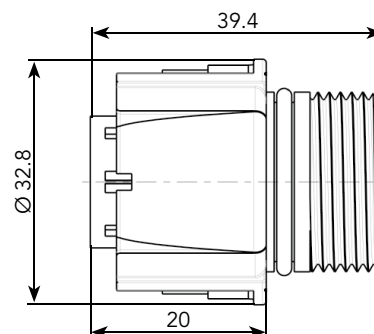
Plug - WME20005A & WME20002A
