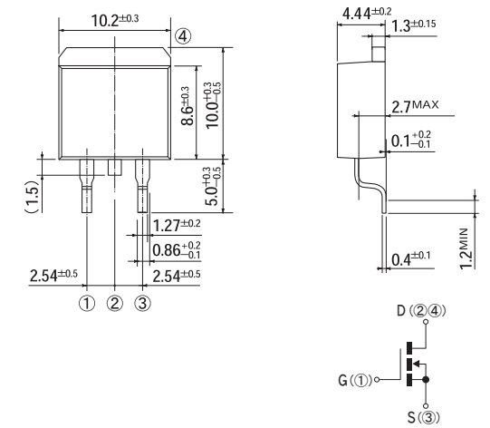
H4 Package: TO-263AB
