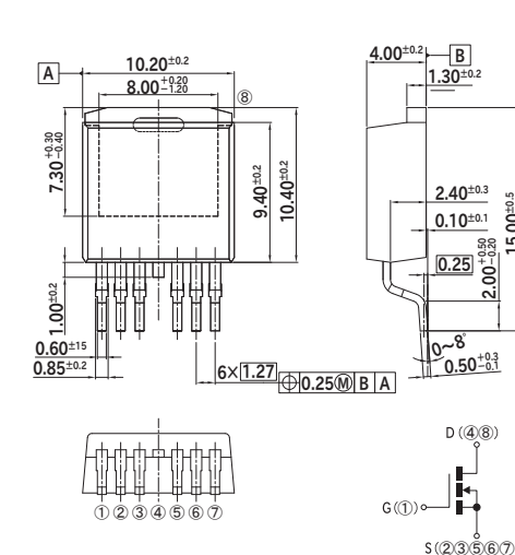
H7 Package: TO-263SC
