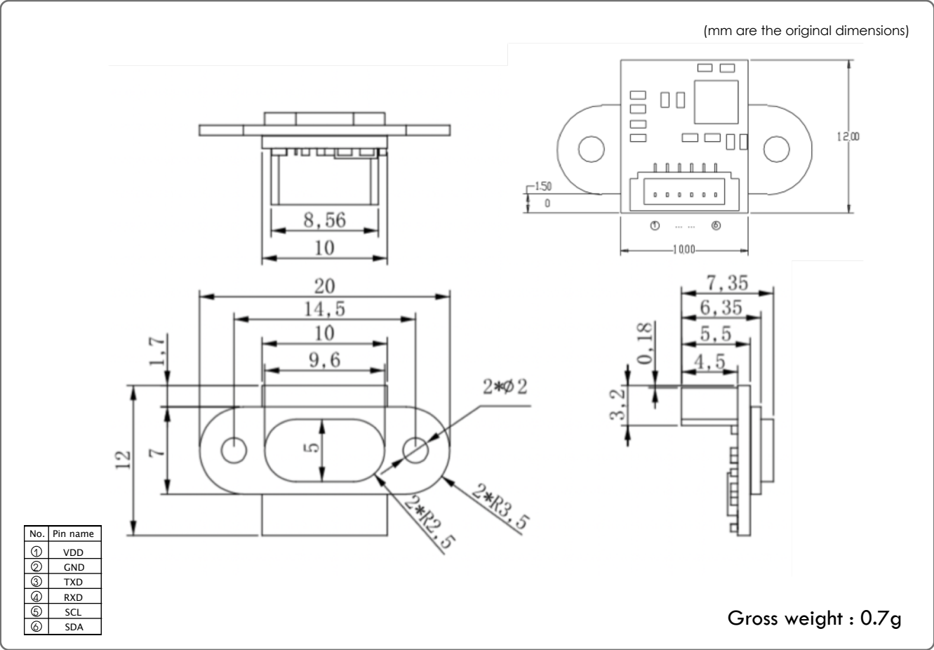
Module OUTLINE
