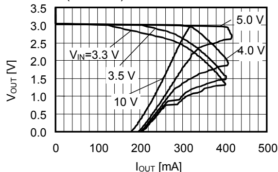
S-L2980A30 (Ta=25°C)
