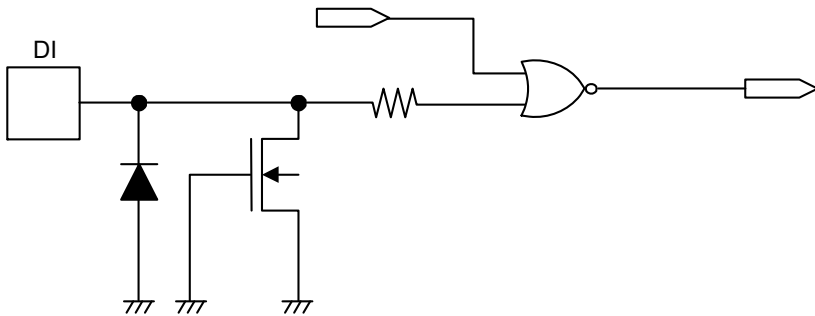
Figure 20 DI Pin
