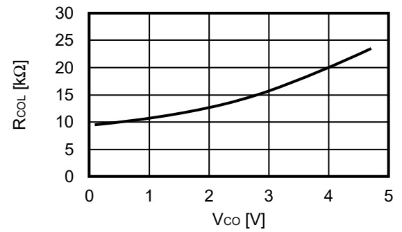
4. 2 R_{COL} vs. V_{CO}
