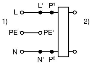
1) Line 2) Load
