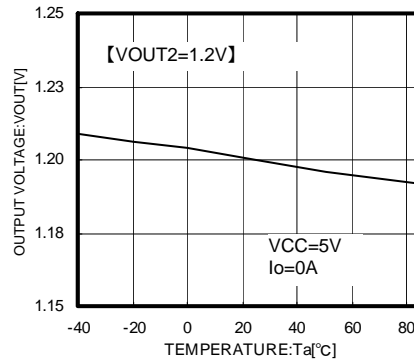
Fig. 7 Ta - VOUT
