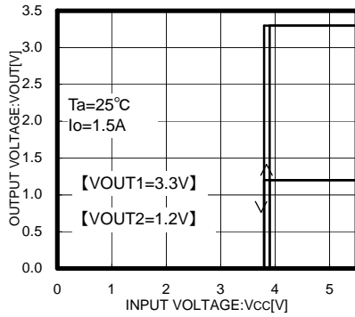
Fig.3 Vcc - VOUT
