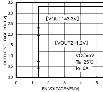
Fig.4 VEN - VOUT
