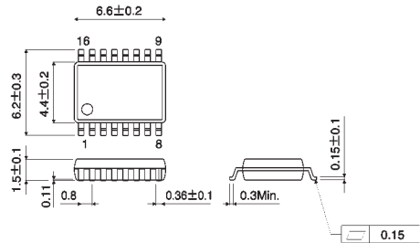
SSOP-A16
