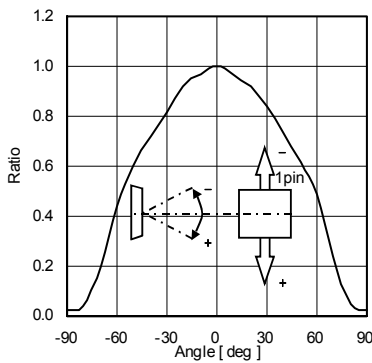
Fig.5 ALS Directional Characteristics 2
