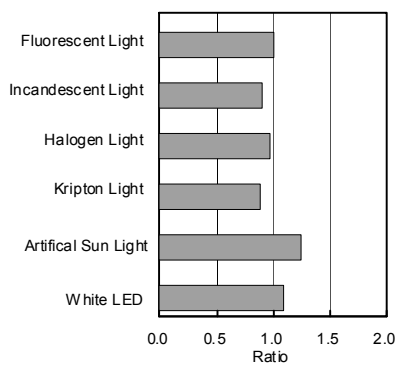
Fig.8 ALS Light Source Dependency ( Fluorescent Light is set to '1' )
