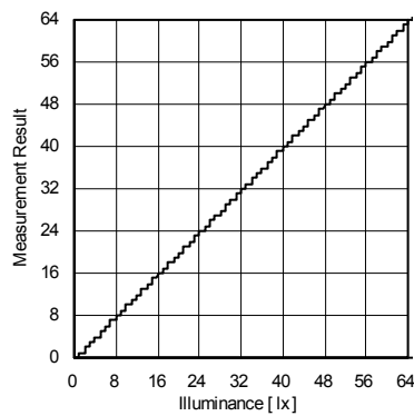
Fig.2 Illuminance - ALS Measuremnet Result
