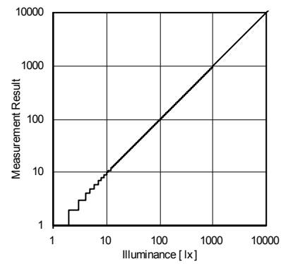
Fig.3 Illuminance - ALS Measuremnet Result 2
