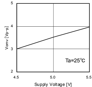
Fig.37 Vomv (PB-13.5MHz)
