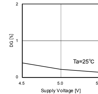
Fig.55 DG(PY-13.5MHz)
