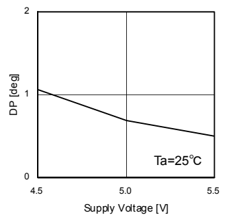
Fig.79 DP(PR-30MHz)
