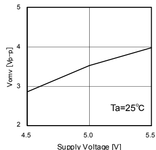
Fig.43 Vomv (PR-30MHz)
