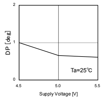
Fig.73 DP(PB-13.5MHz)
