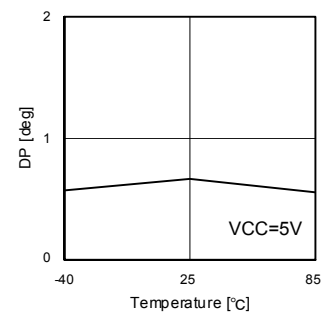
Fig.76 DP(PR-13.5MHz)
