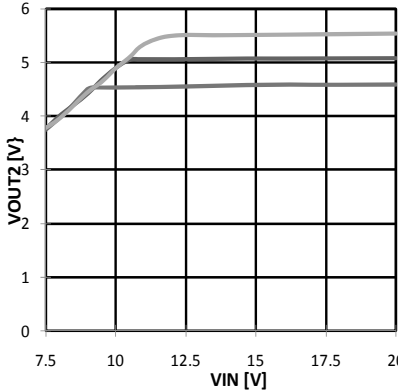
Fig.18 VIN-VOUT2
