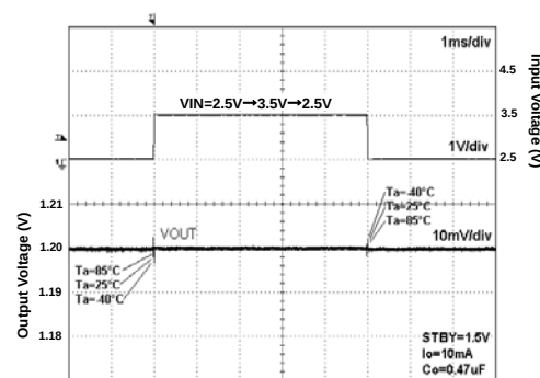
Fig 27. VIN Response
