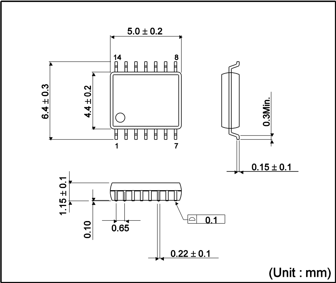
SSOP-B14
