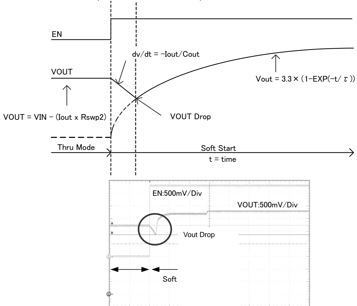
Figure 47. EN : L=>H PFM I_o=5mA VIN=3.6V
