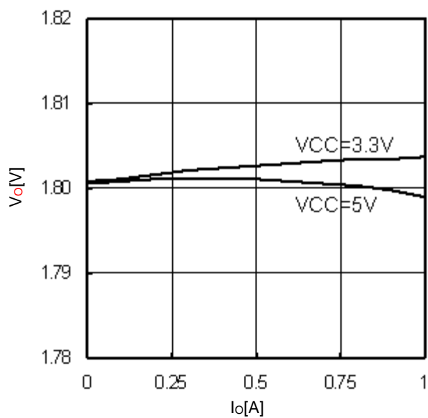
Fig.17 Io-Vo (Vo=1.8V)
