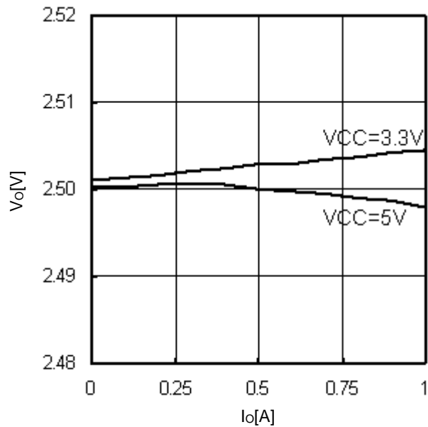
Fig.18 Io-Vo (Vo=2.5V)
