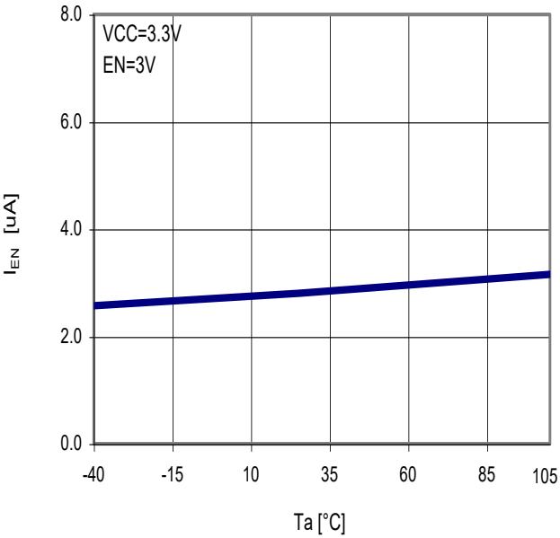
Fig.24 T_a - I_{EN}
