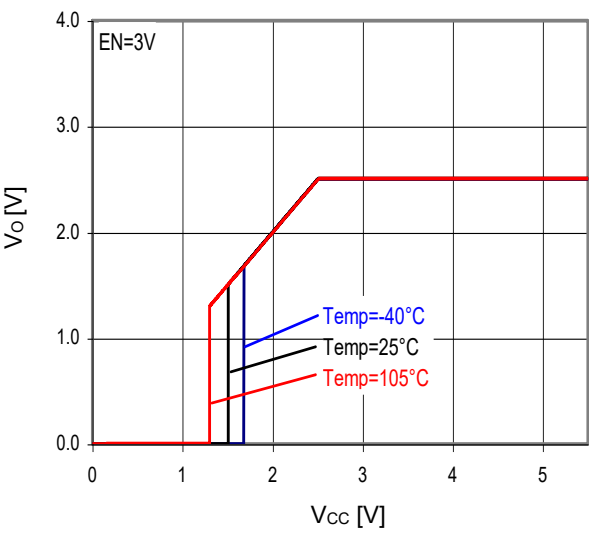
Fig.27 V_{cc}-V_o ( I_o=0\text{mA} )
