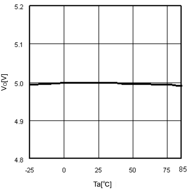
Fig.9 Ta-Vo (Io=0mA)
