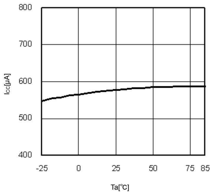
Fig.10 Ta-Icc
