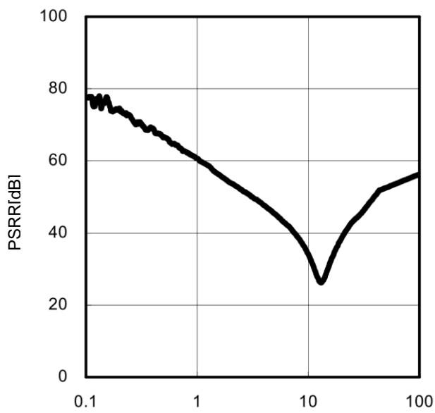
Fig.33 PSRR( I_o=0mA )
