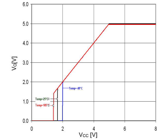
Fig.27 Vcc-Vo (Io=0mA)
