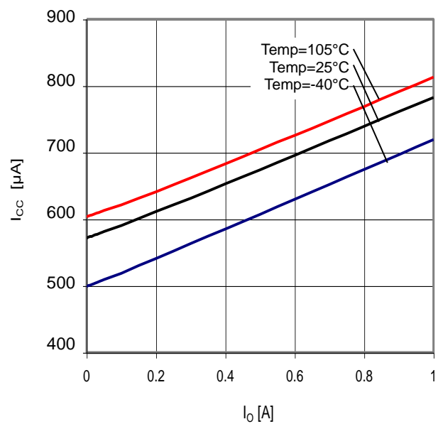
Fig.30 I_o-I_{cc}
