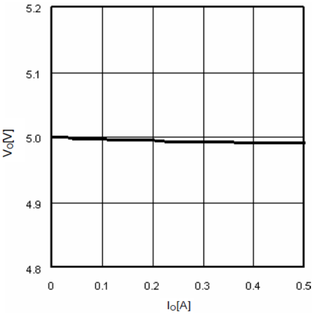
Fig. 25 I_O - V_O
