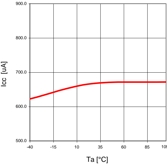
Fig.22 T_a-I_{CC}
