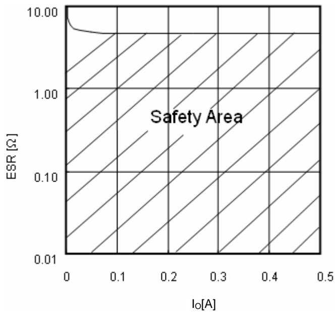
Fig.19 ESR condenser
