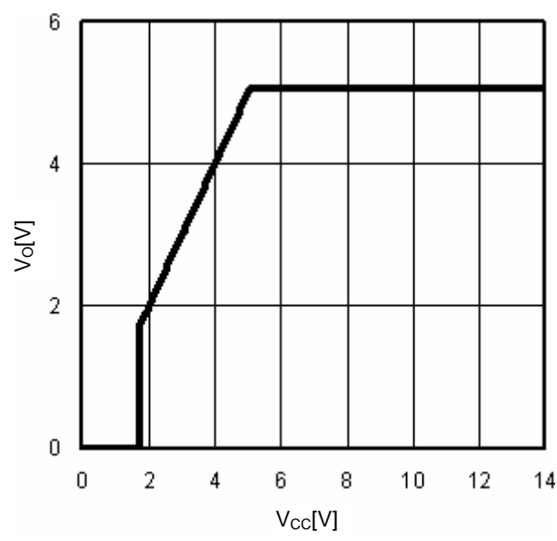
Fig.15 V_{CC}-V_O ( I_O=0mA )
