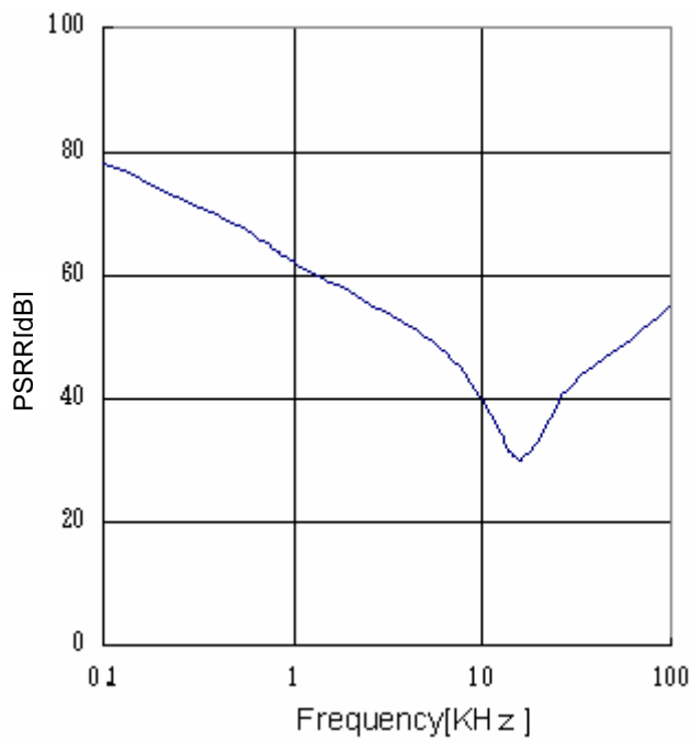
Fig.21 PSRR ( I_o=0\text{mA} )
