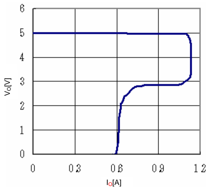
Fig.17 OCP
