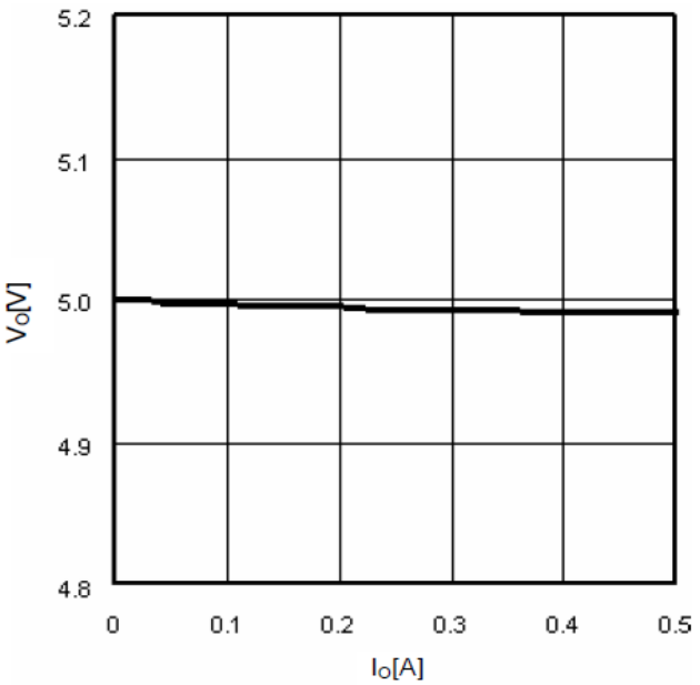
Figure 25. I O -V O
