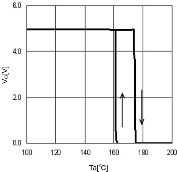
Figure 28. TSD ( I_O=0\text{mA} )
