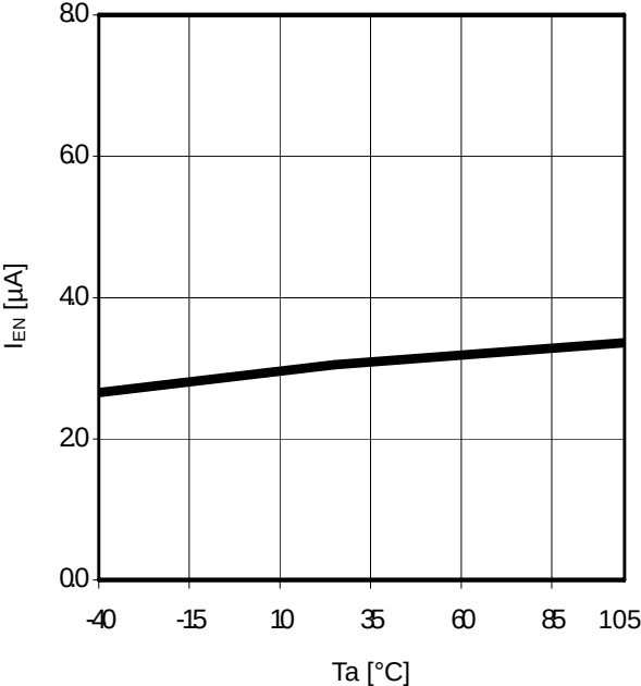
Figure 24. Ta-I EN
