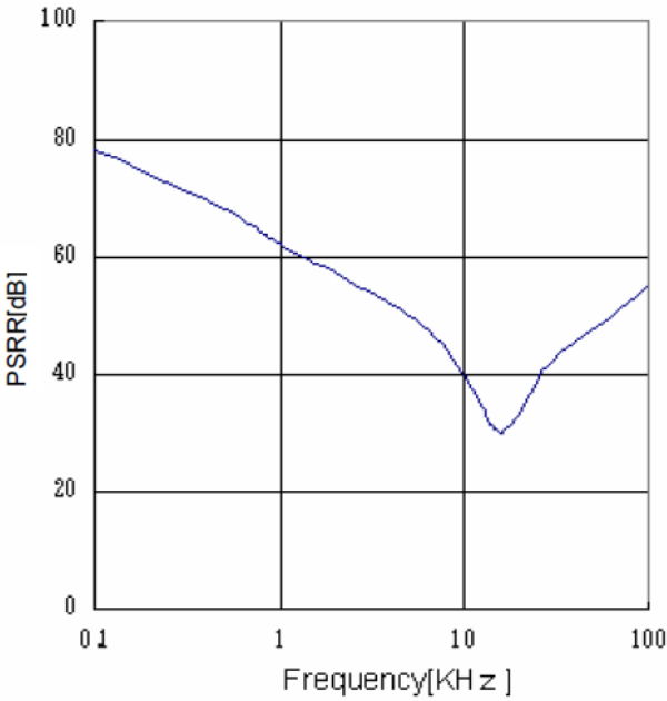
Figure 32. PSRR (I_o=0mA)
