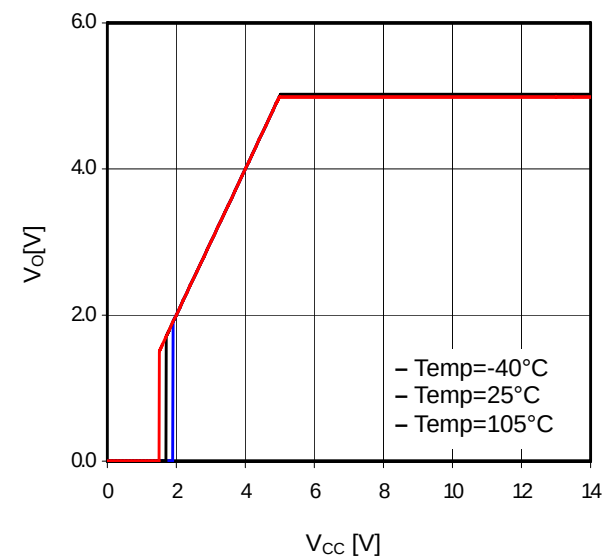
Figure 27. V_{CC}-V_O ( I_O=0\text{mA} )
