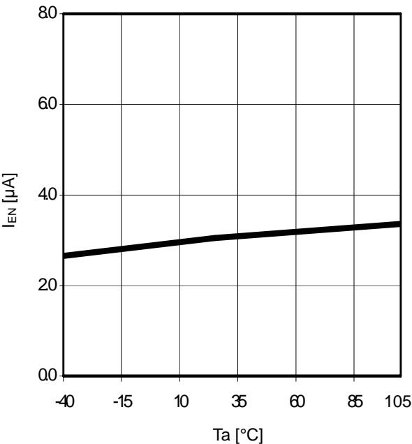
Fig. 24 T_a - I_{EN}
