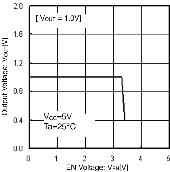
Figure 6. Output Voltage vs EN Volatge
