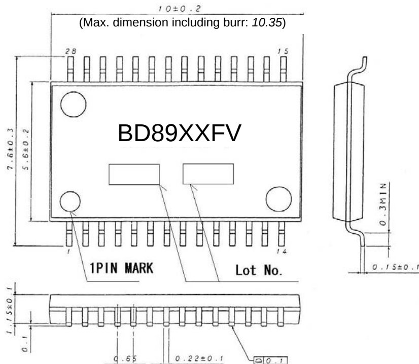
Fig. 5 SSOP-B28 Package Outer Dimension
