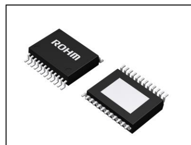
HTSSOP-B24
