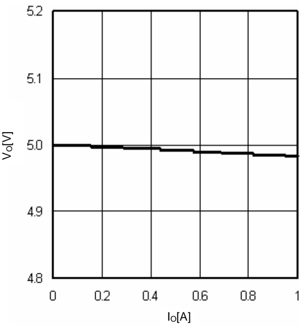
Fig.12 I_O - V_O
