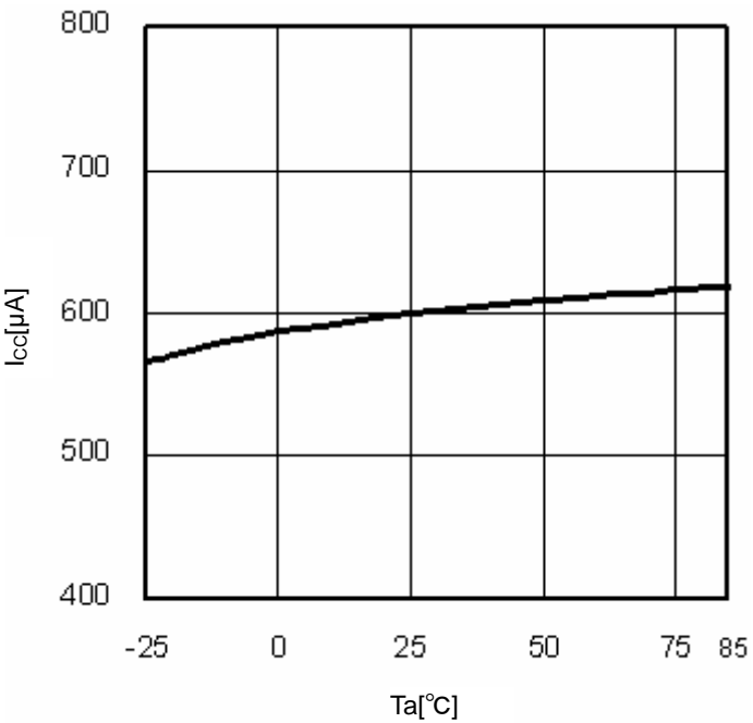
Fig.9 T_a-I_{cc}
