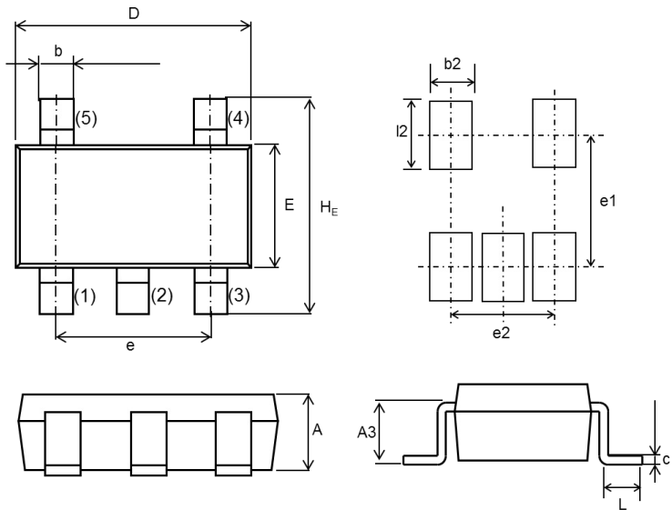
SOT-25T, (TSMD5)
