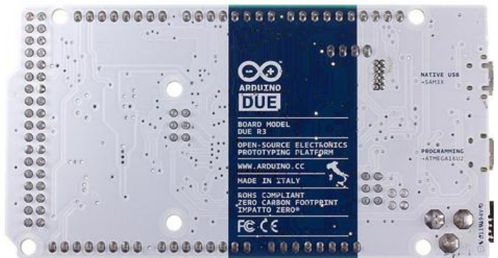
Arduino Due Back
