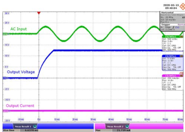
CH2: V_{IN} , 500 V / div., 10 ms / div. CH3: V_{OUT} , 5 V / div., 10 ms / div. CH4: I_{OUT} , 250 mA / div., 10 ms / div. Rise Time = 6.6378 ms.
