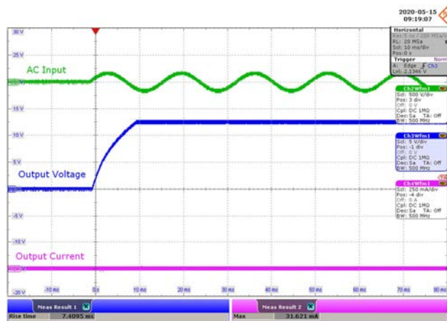
CH2: V_{IN} , 500 V / div., 10 ms / div. CH3: V_{OUT} , 5 V / div., 10 ms / div. CH4: I_{OUT} , 250 mA / div., 10 ms / div. Rise Time = 7.4095 ms.
