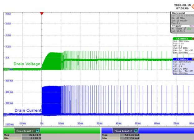
CH2: V_{DS} , 200 V / div., 10 ms / div. CH3: I_{DS} , 200 mA / div., 10 ms / div. V_{DS(MAX)} = 324.11 V. I_{DS(MAX)} = 515.42 mA.
