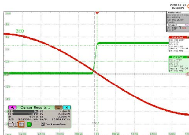
CH1: V_{IN} , 100 V / div., 800 \mu s / div. CH2: ZCD, 2 V / div., 800 \mu s / div. Falling edge delay = -104 \mu s.
