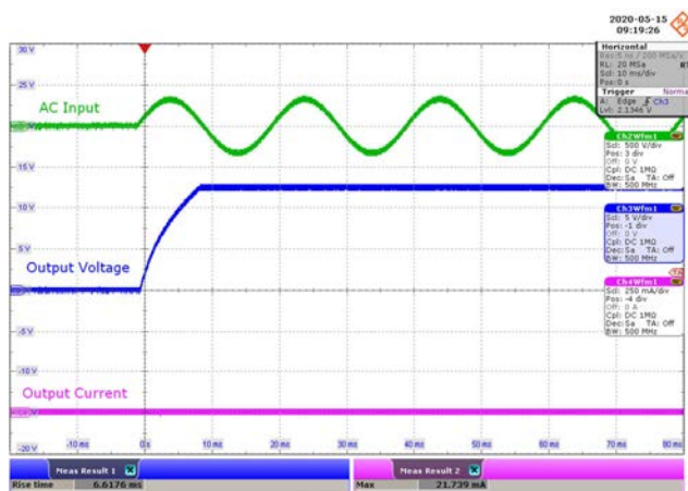
CH2: V_{IN} , 500 V / div., 10 ms / div. CH3: V_{OUT} , 5 V / div., 10 ms / div. CH4: I_{OUT} , 250 mA / div., 10 ms / div. Rise Time = 6.6176 ms.
