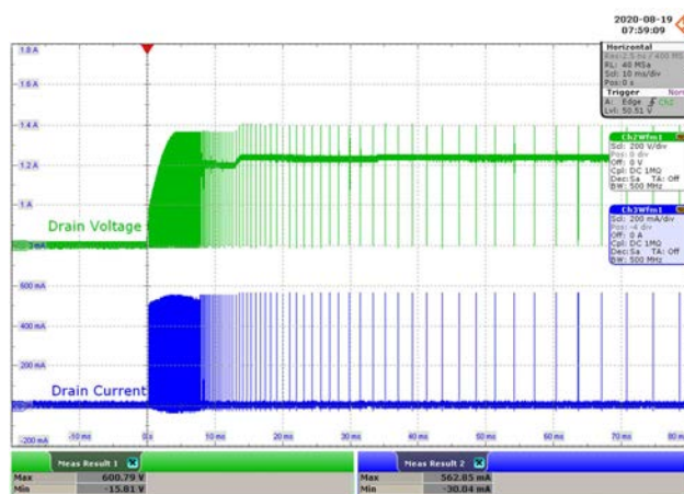
CH2: V_{DS} , 200 V / div., 10 ms / div. CH3: I_{DS} , 200 mA / div., 10 ms / div. V_{DS(MAX)} = 600.79 V. I_{DS(MAX)} = 562.85 mA.
