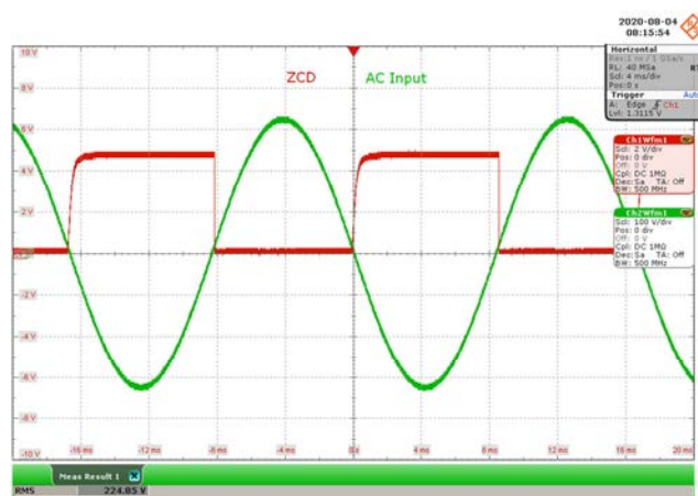
CH1: ZCD, 2 V / div., 4 ms / div. CH2: V_{IN} , 100 V / div., 4 ms / div.
