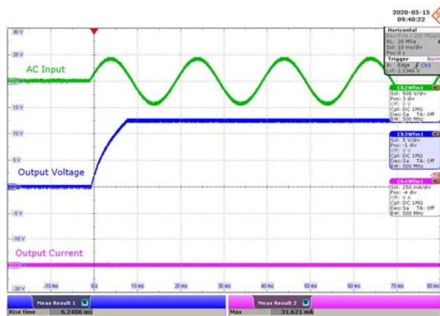
CH2: V_{IN} , 500 V / div., 10 ms / div. CH3: V_{OUT} , 5 V / div., 10 ms / div. CH4: I_{OUT} , 250 mA / div., 10 ms / div. Rise Time = 6.2406 ms.
