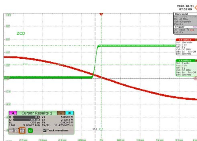
CH1: V_{IN} , 100 V / div., 800 \mu s / div. CH2: ZCD, 2 V / div., 800 \mu s / div. Rising edge delay = -256 \mu s.
