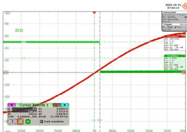
CH1: V_{IN} , 100 V / div., 800 \mu s / div. CH2: ZCD, 2 V / div., 800 \mu s / div. Falling edge delay = 240 \mu s.
