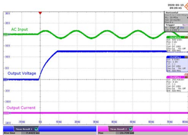
CH2: V_{IN} , 500 V / div., 10 ms / div. CH3: V_{OUT} , 5 V / div., 10 ms / div. CH4: I_{OUT} , 250 mA / div., 10 ms / div. Rise Time = 7.4422 ms.
