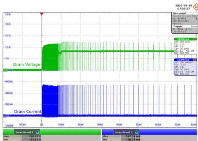
CH2: V_{DS} , 200 V / div., 10 ms / div. CH3: I_{DS} , 200 mA / div., 10 ms / div. V_{DS(MAX)} = 498.02 V. I_{DS(MAX)} = 547.04 mA.
