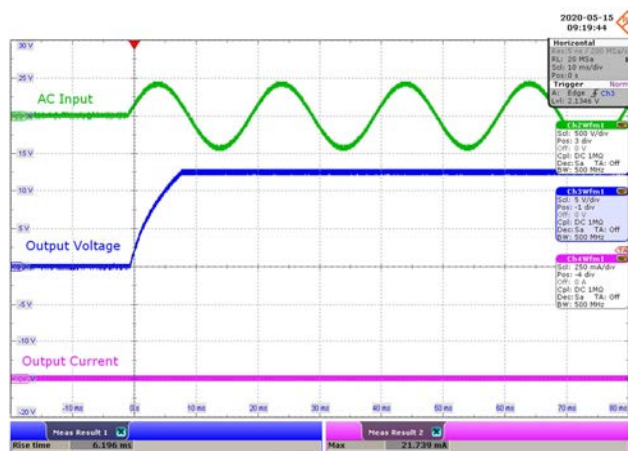
CH2: V_{IN} , 500 V / div., 10 ms / div. CH3: V_{OUT} , 5 V / div., 10 ms / div. CH4: I_{OUT} , 250 mA / div., 10 ms / div. Rise Time = 6.196 ms.
